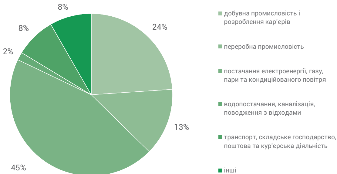
Рис. 27. Структура викидів в атмосферне повітря Харківської області за джерелами забруднення у 2018 р.
